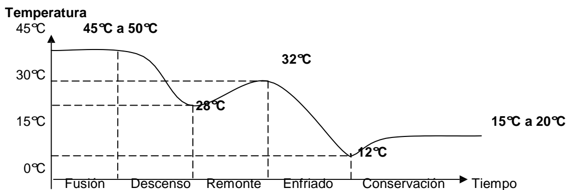
Típica curva de templado de un chocolate
